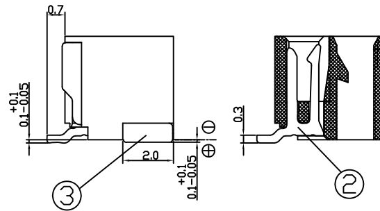
剖面 A-A
